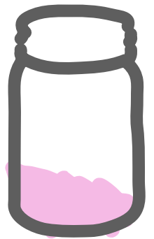
skin
