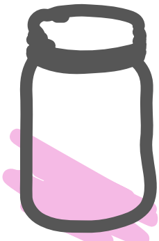
eyes
